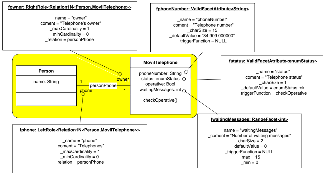
Figura 3: Ejemplo con metainformaciones
