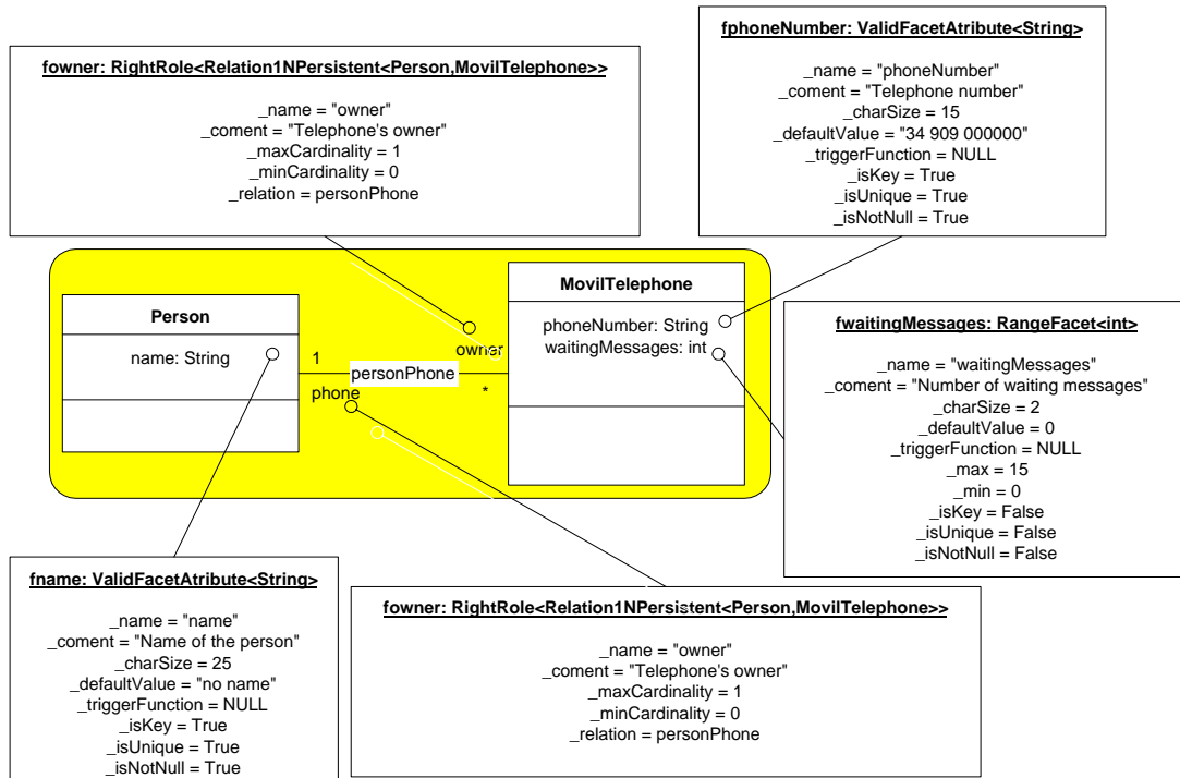
Figura 4: Ejemplo de aplicación
