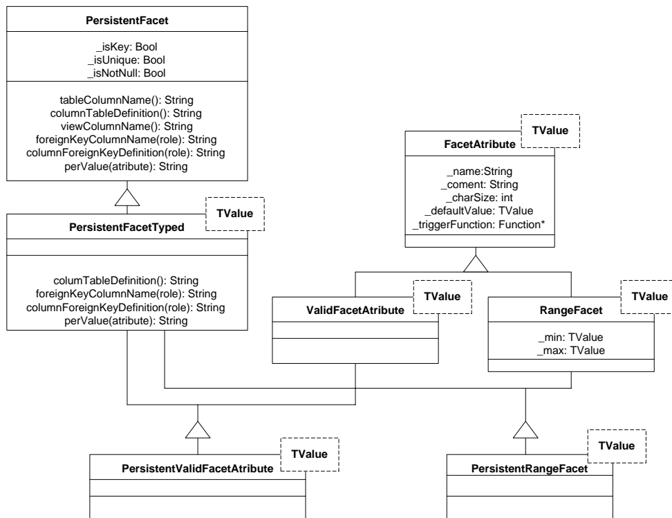
Figura 2: Jerarquía de facets
