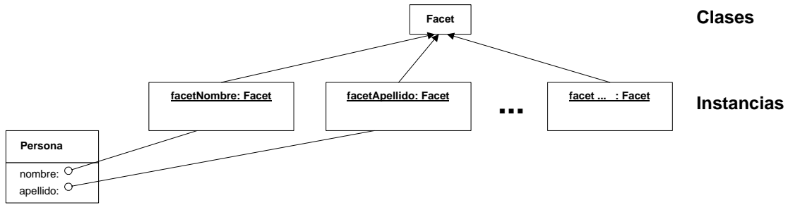
Figura 1: Estructura a tres niveles (objeto-slot-facet).
